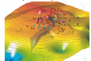
Поверхность кровли пласта
