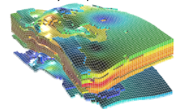
Поверхность кровли пласта
